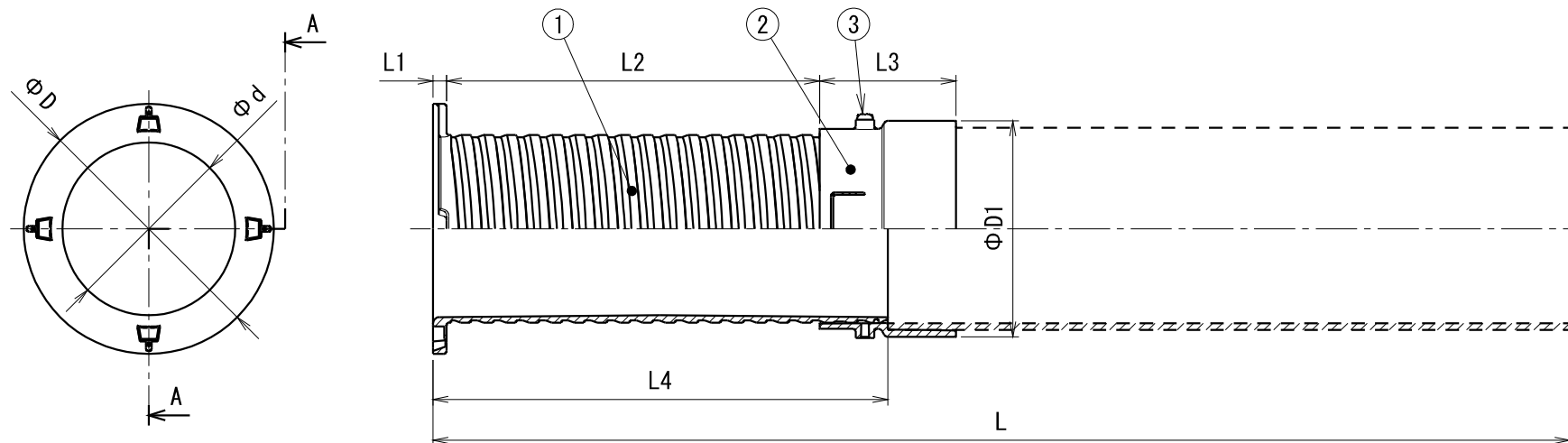
断面 A-A
